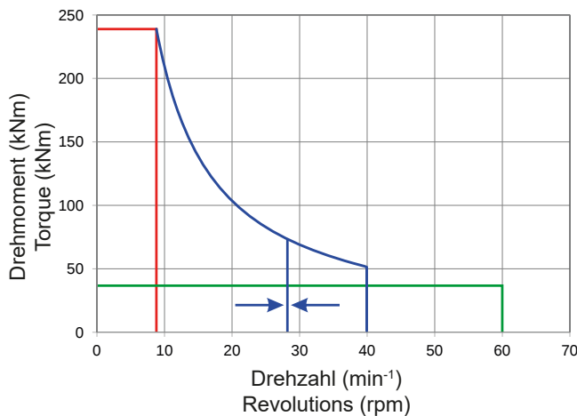
Kellybohrantrieb BT 240 / Rotary Head BT 240
